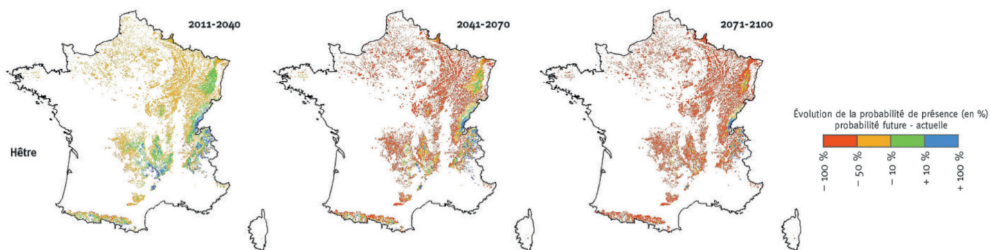
Figure 4. Evolution de la probabilité de présence du hêtre dans le futur pour 3 périodes de référence : 2011-2040, 2041-2070, 2071-2100.
